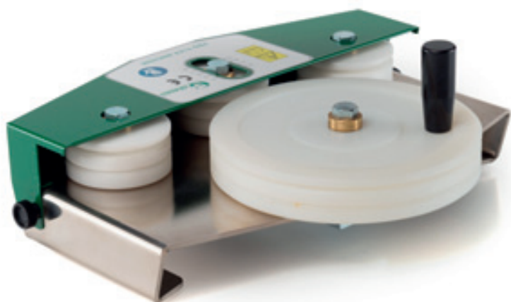
PROFLEX MACHINE - macchina manuale per curvare i profili proflex line
